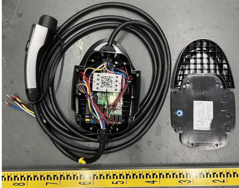
内部结构
