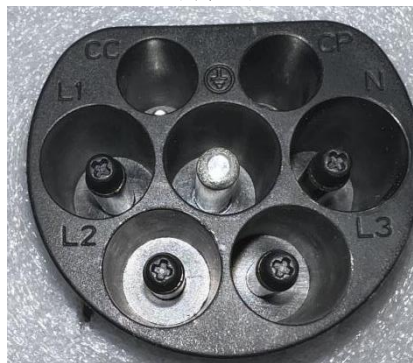
插合面
