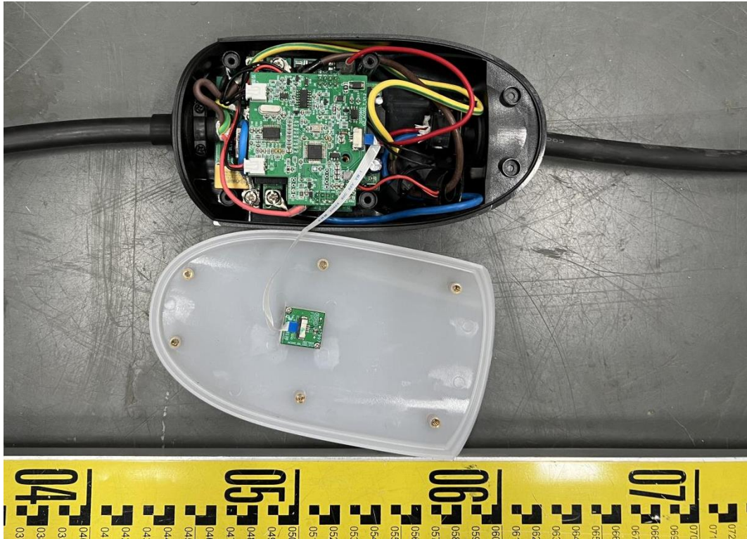
内部结构
